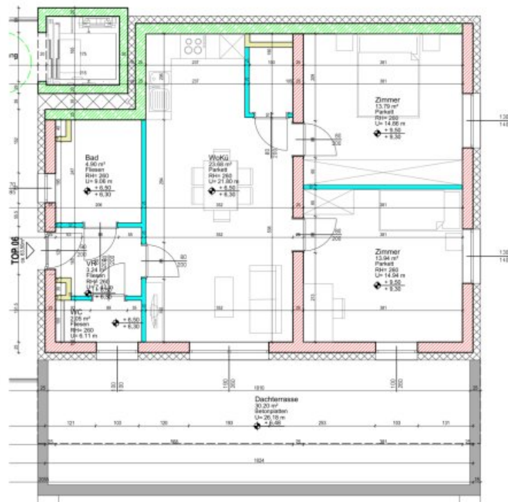
Planausschnitt 3.OBERGESCHOSS - Wohnung
