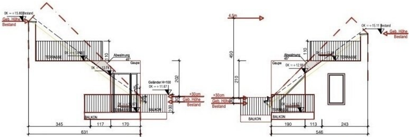
Ansicht 2 Hoftrakt
