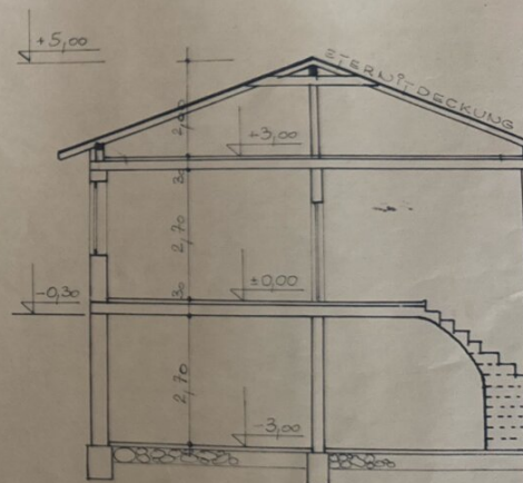
SCHNITT
