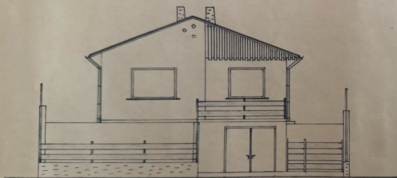
STRASSENANSICHT
