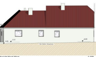
Ansicht Nord-West 1:100
