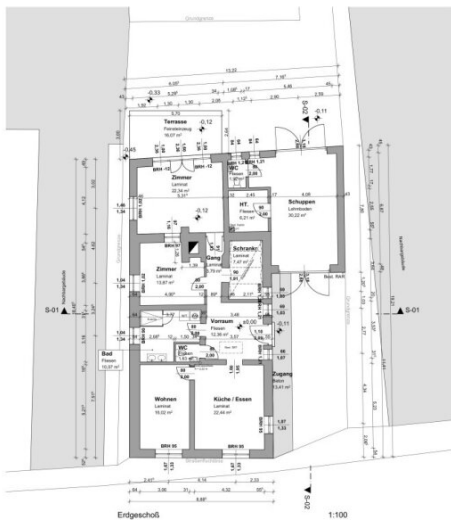
Erdgeschoss 1:100
