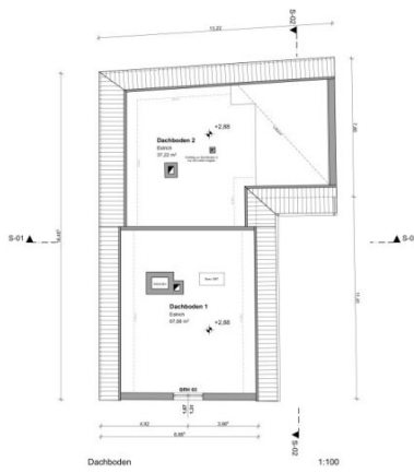
Dachboden 1:100
