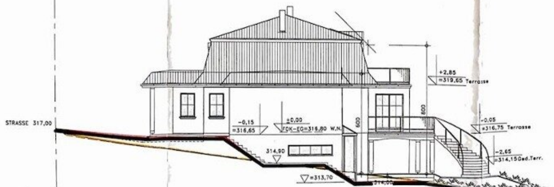
WEST-ANSICHT
