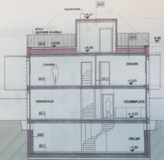
SCHNITT 1-1
