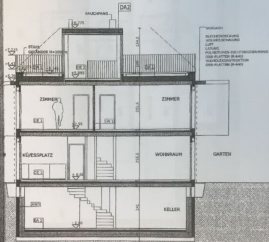
SNITT 1-1
