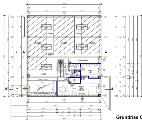
Grundriss OG
