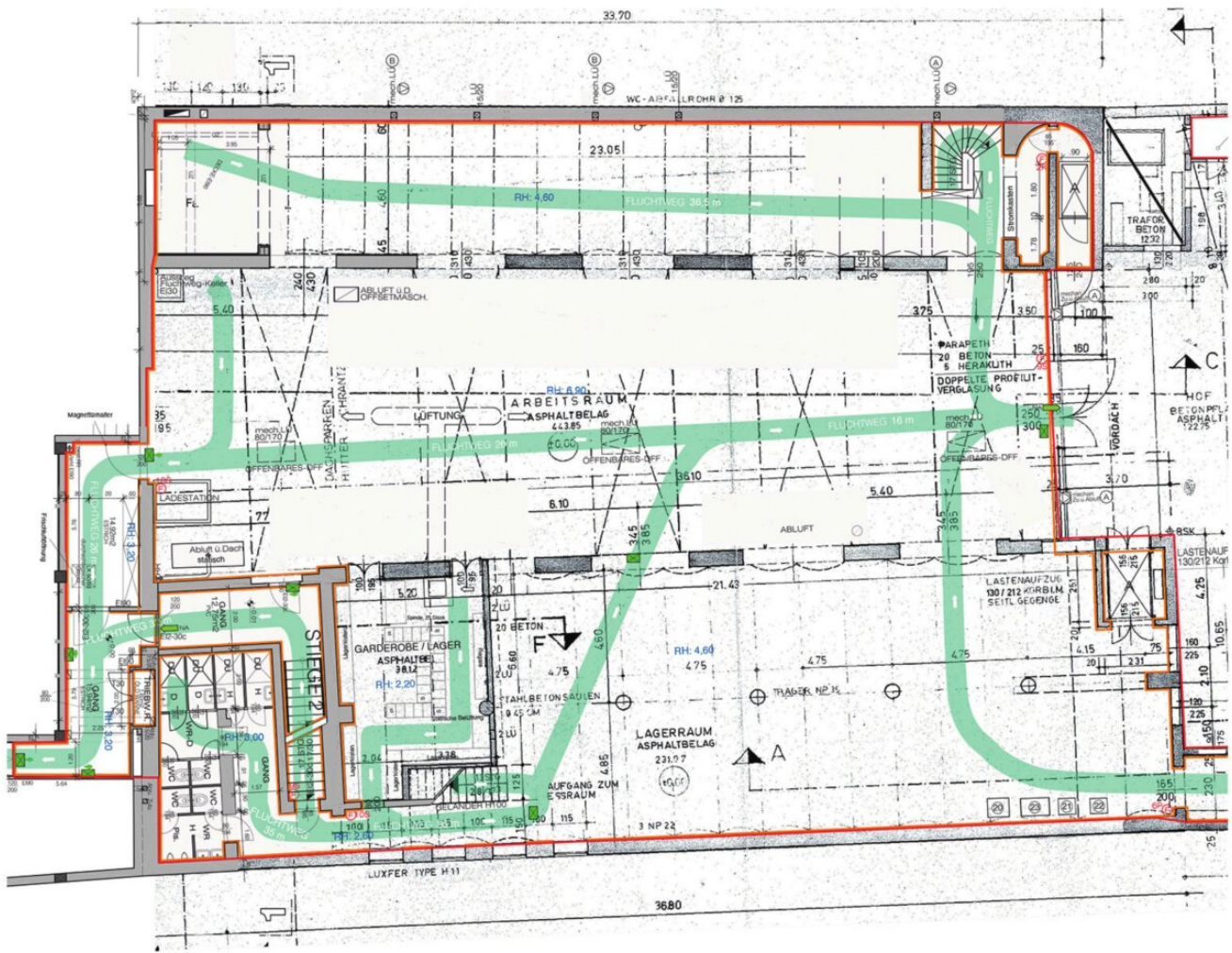
ERDGESCHOSS M 1:100
