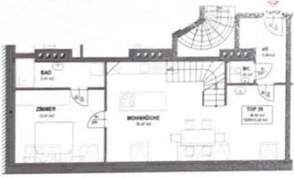
1. Dachgeschoss
