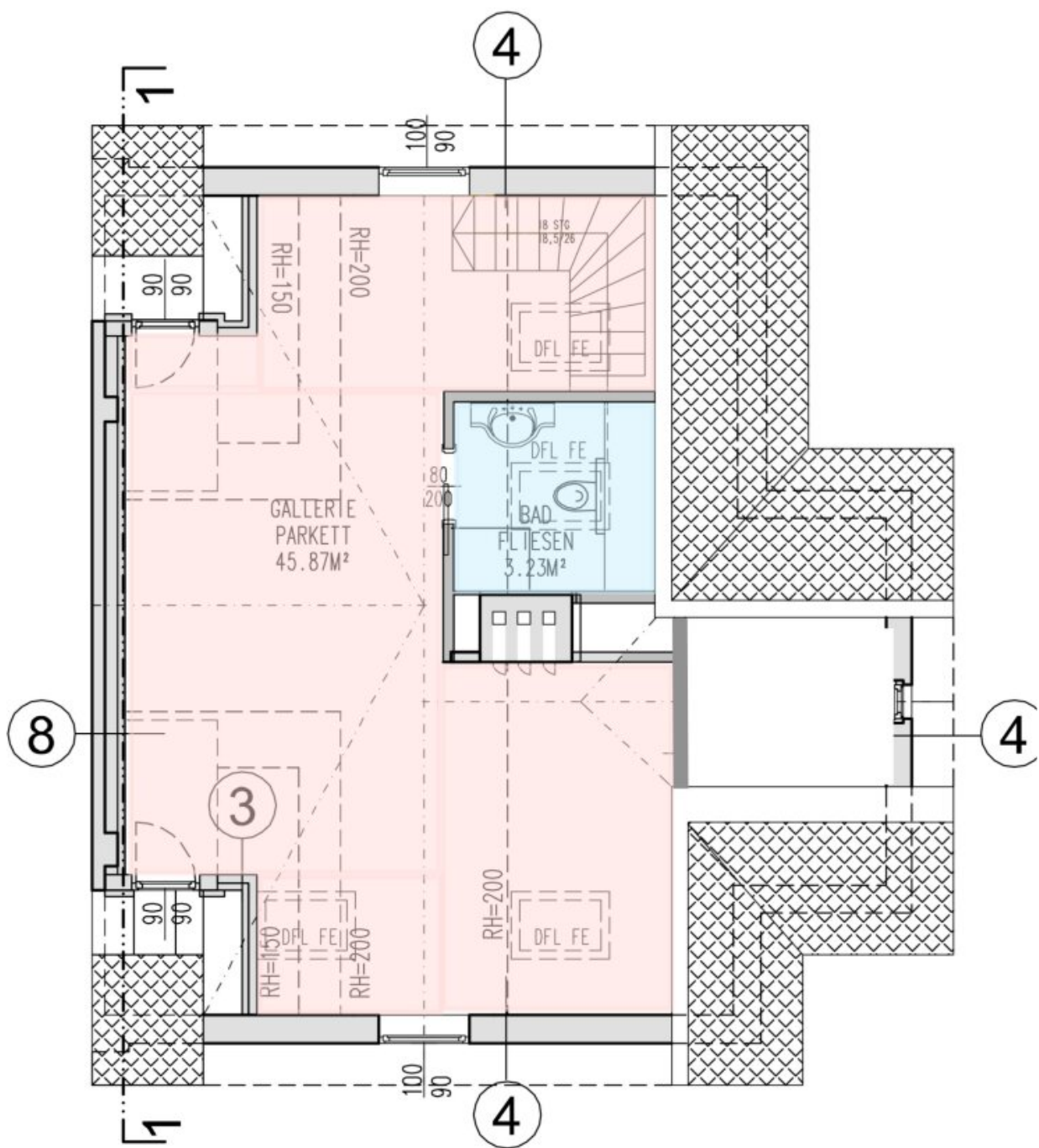
DACHGESCHOSS
