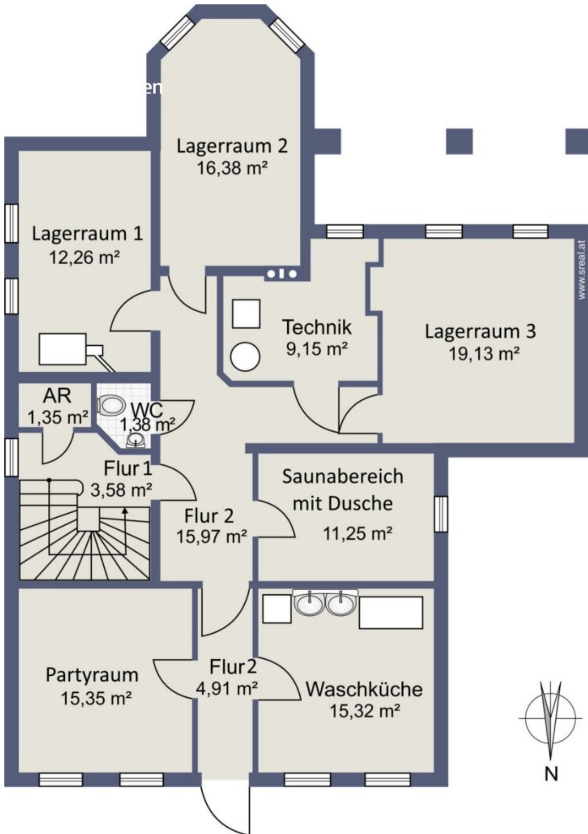
Planskizze Untergeschoss
