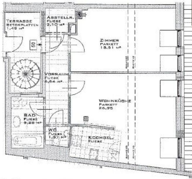
1. DACHGESCHOSS
