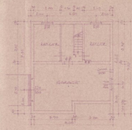
2. Etage
