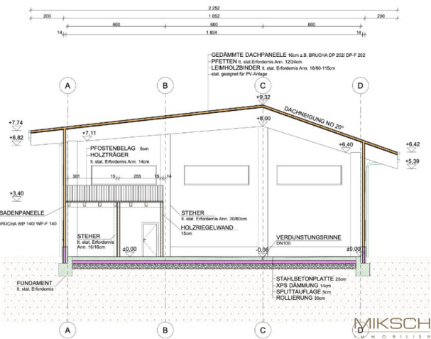
SNITT A-A:
