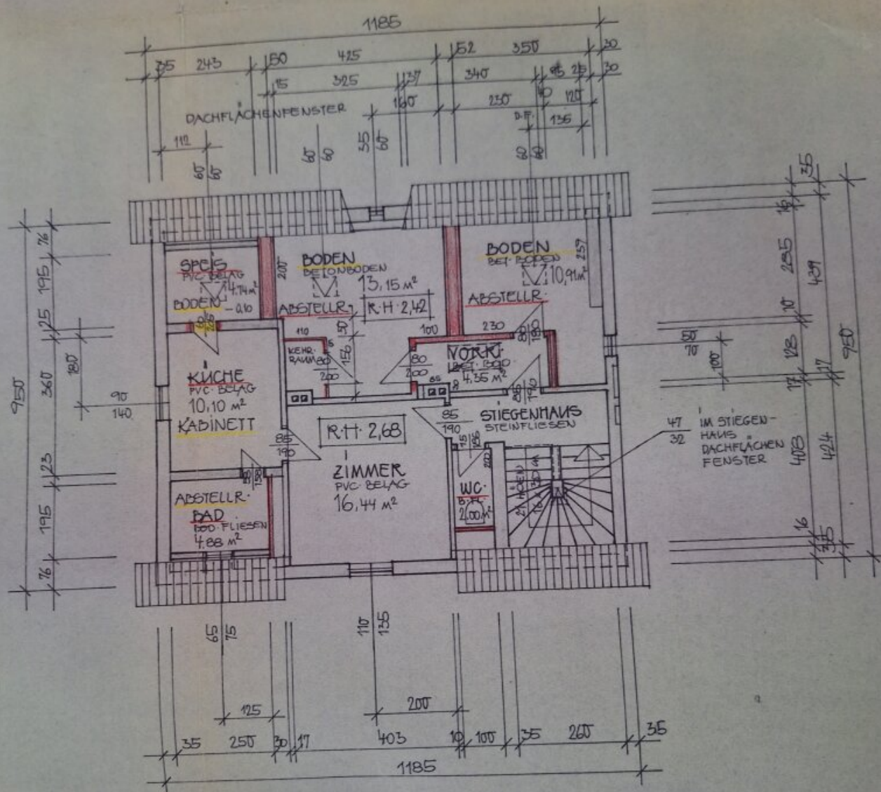
DACHGESCHOSSGRUNDRISS
