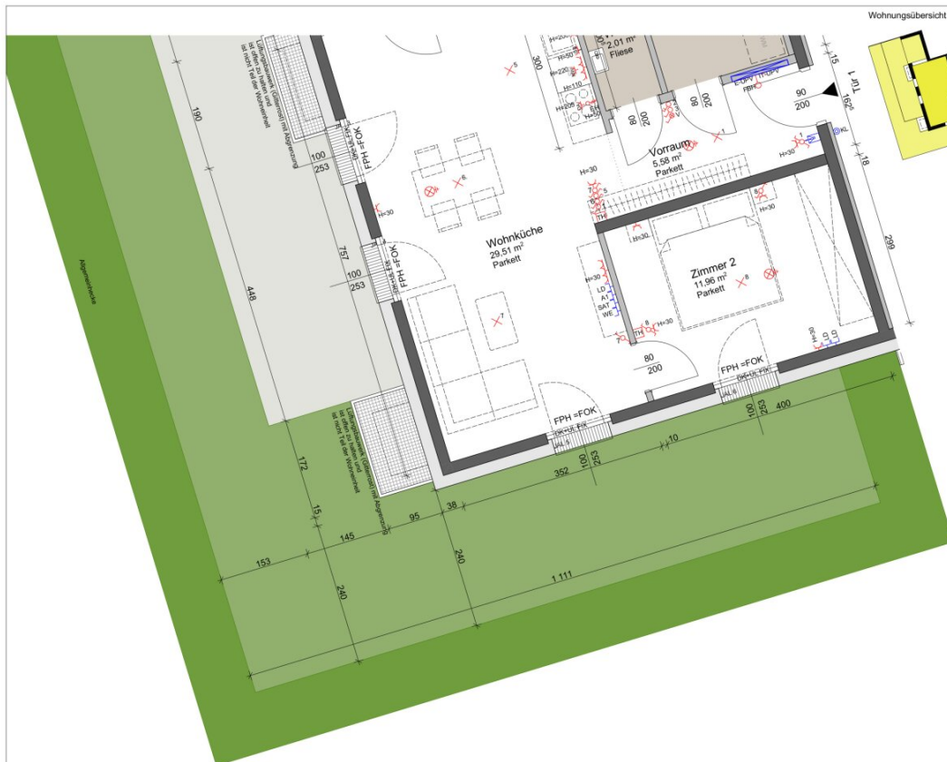
Wohnungsübersicht
