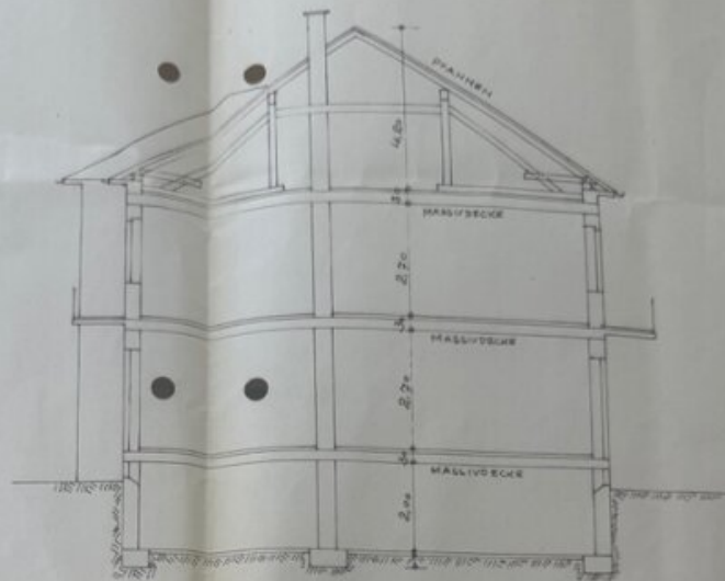
SCHNITT A-B
