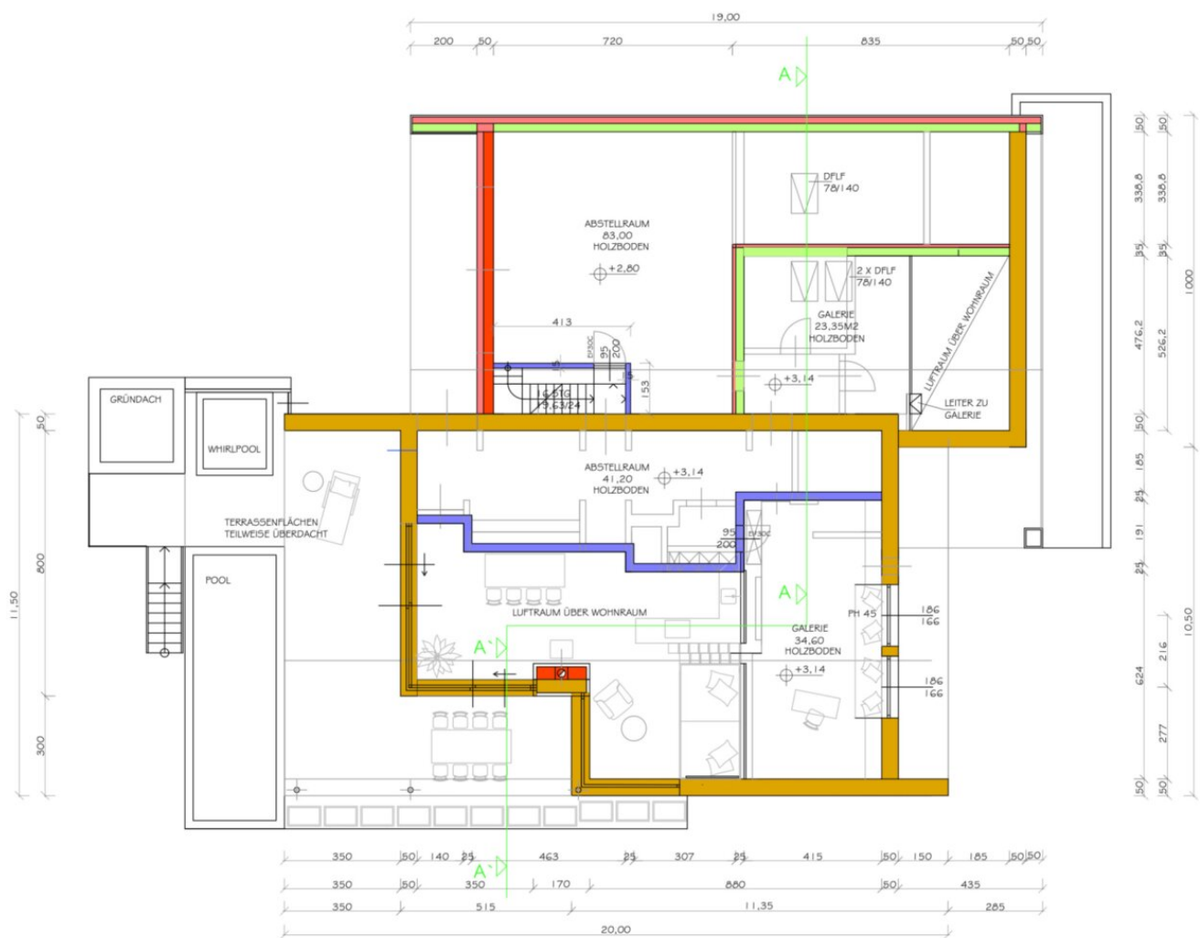
GRUNDRISS AR IM OBERGESCHOSS M 1:100
