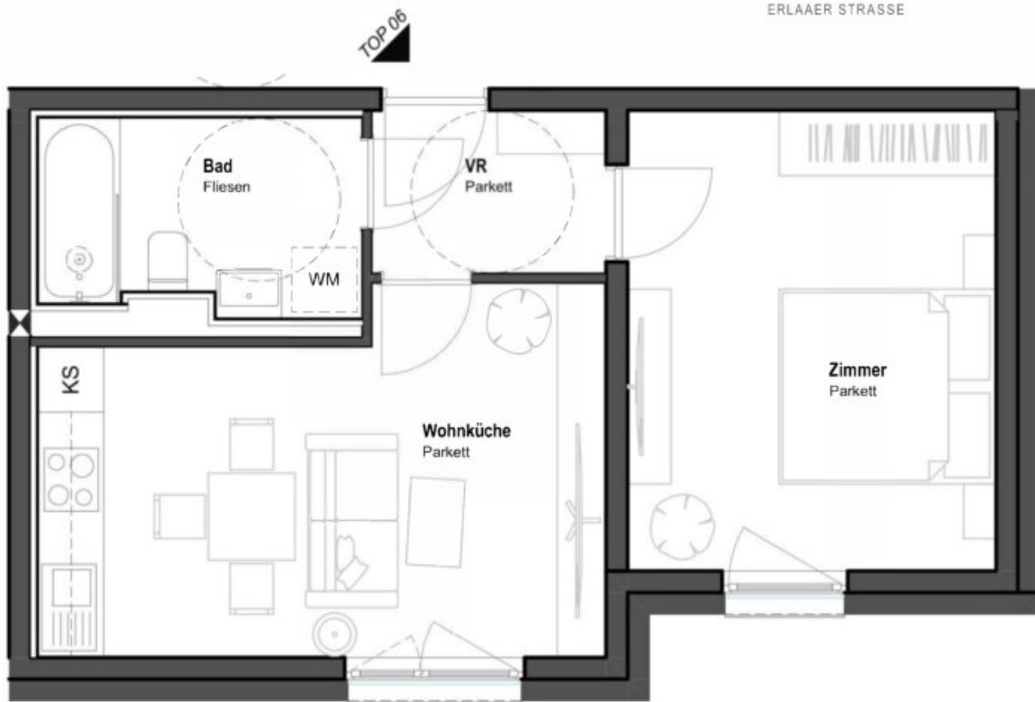
Grundriss 1:50
