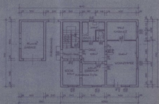
ERDGESCHOSS
