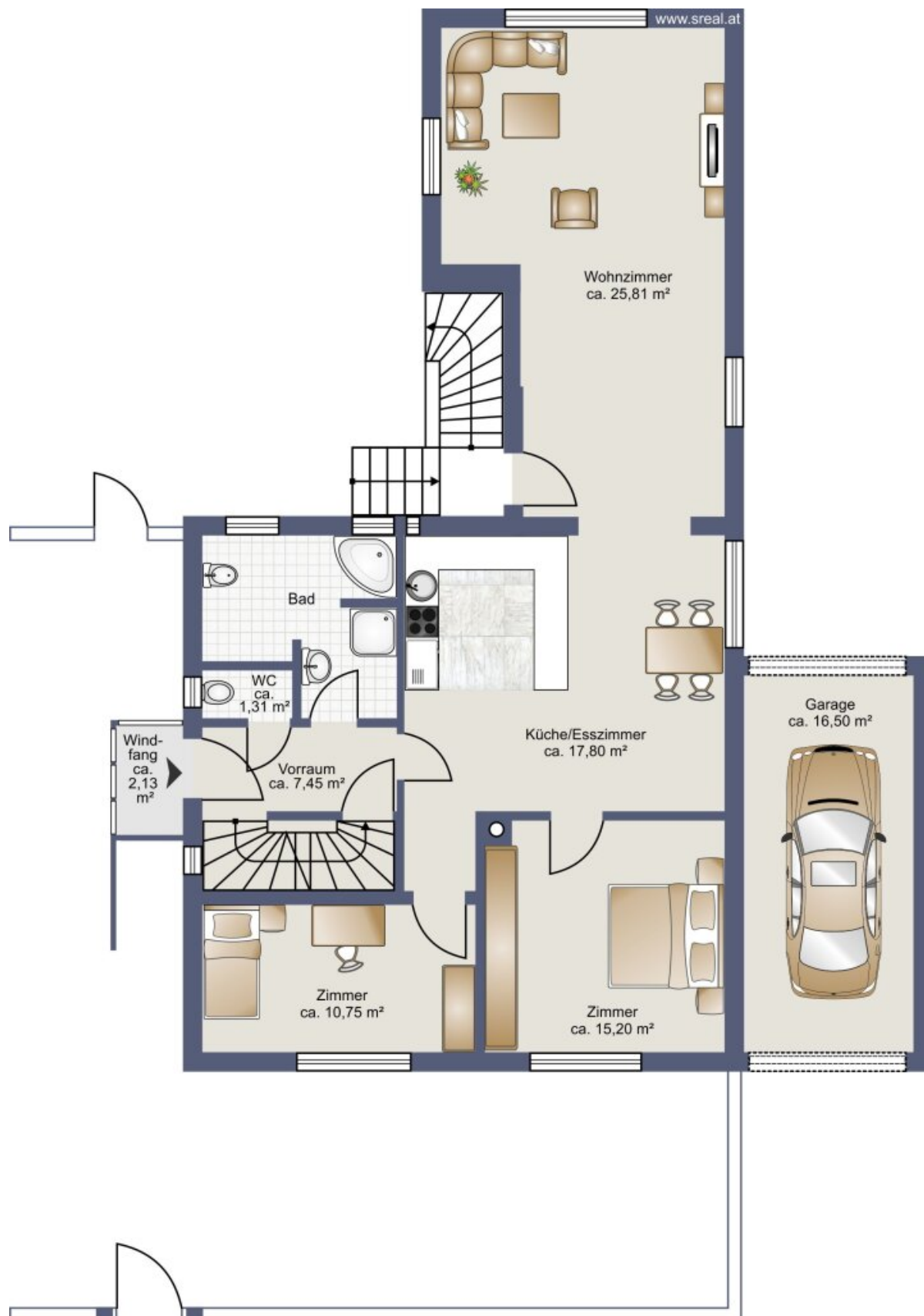
Skizze Erdgeschoss
