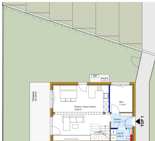
ERDGESCHOSS
