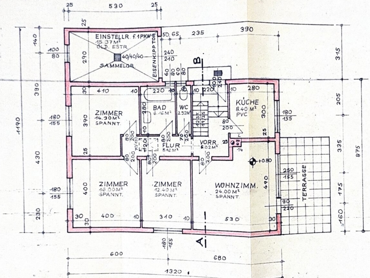
ERDGESCHOSS M=1:100
