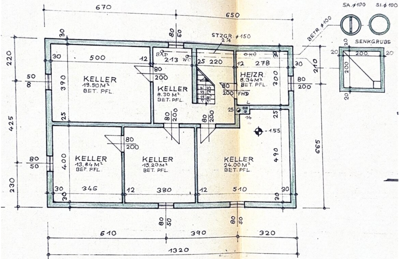
KELLERGESCHOSS M=1:100
