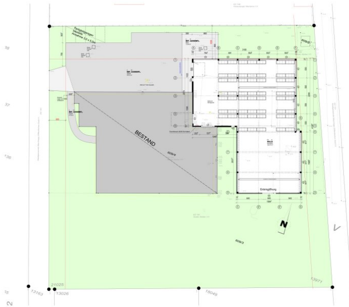
GRUNDRISS ERDGESCHOSS
