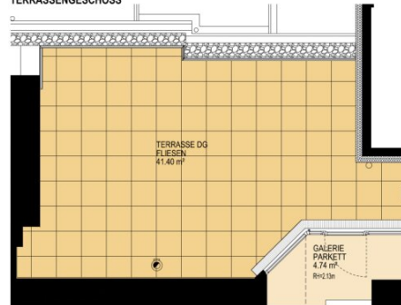
TERRASSENGESCHOSS
