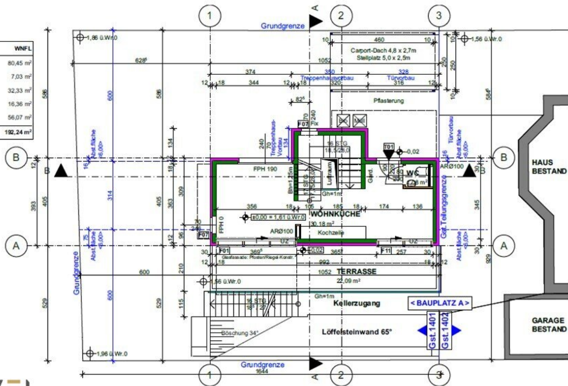
ERDGESCHOSS
