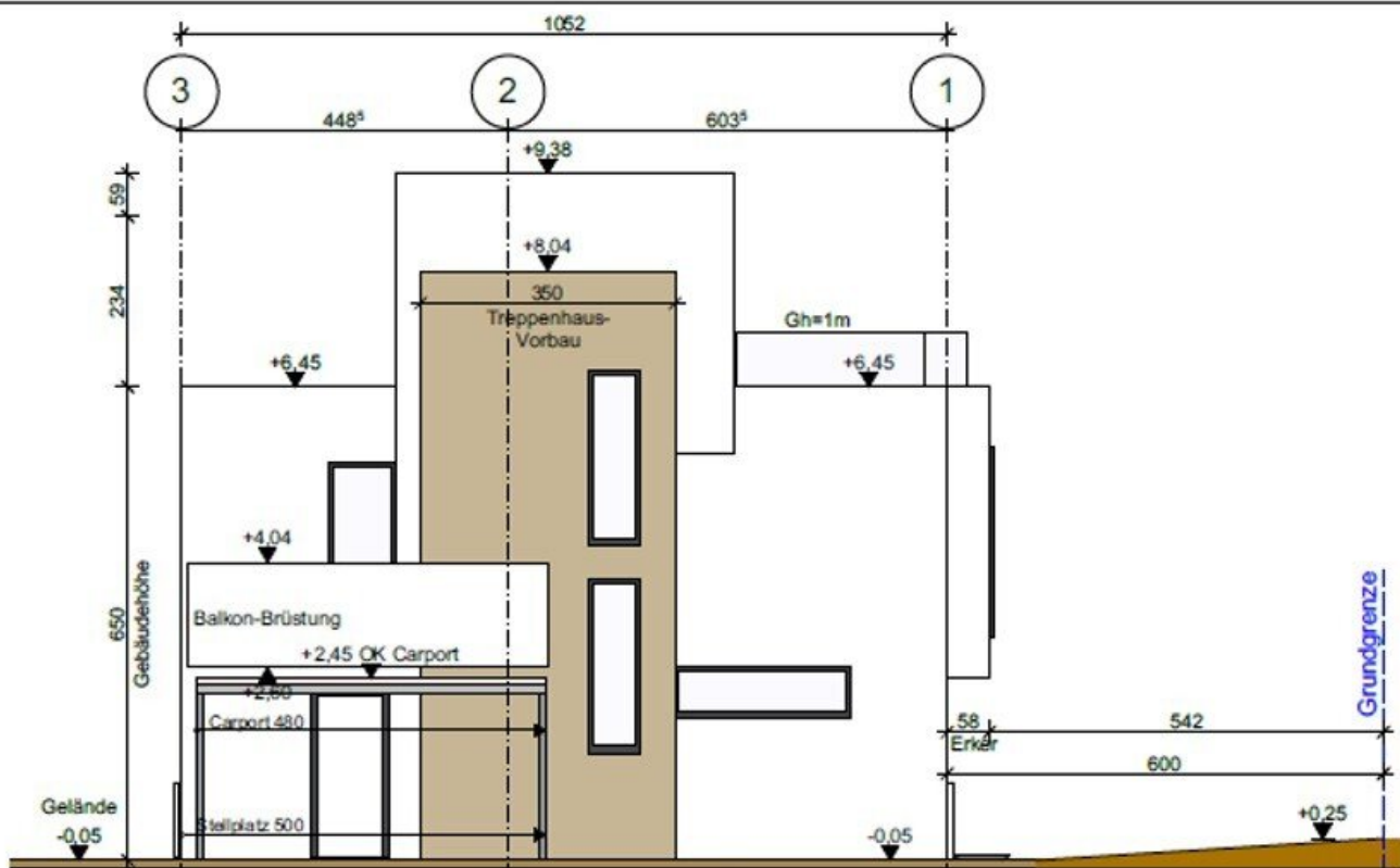
NORDANSICHT
