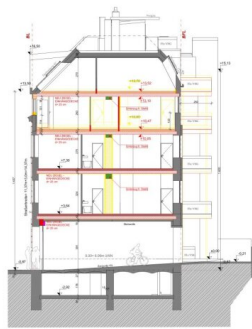
SCHNITT 3-3
