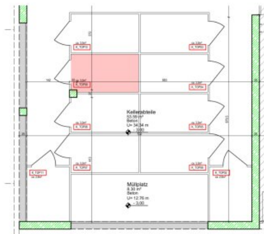
Planausschnitt KELLERGECHOSS - Abteil TOP 09 - OST Planstand = Ausführungsplan M: 1:100
