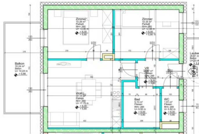
Planausschnitt 3.OBERGESCHOSS - Wohnung Planstand = Ausführungsplan M: 1:100
