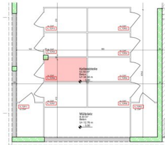
Planausschnitt KELLERGESCHOSS - Abteil TOP 08 - OST Planstand = Ausführungsplan M: 1:100
