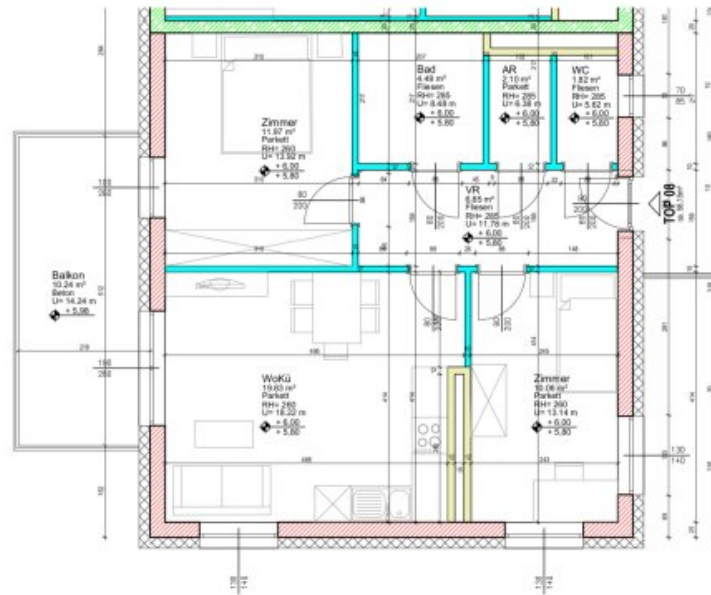
Planausschnitt 3.OBERGESCHOSS - Wohnung Planstand = Ausführungsplan M: 1:100
