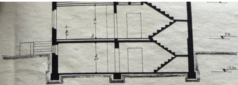
SCHNITT A-B
