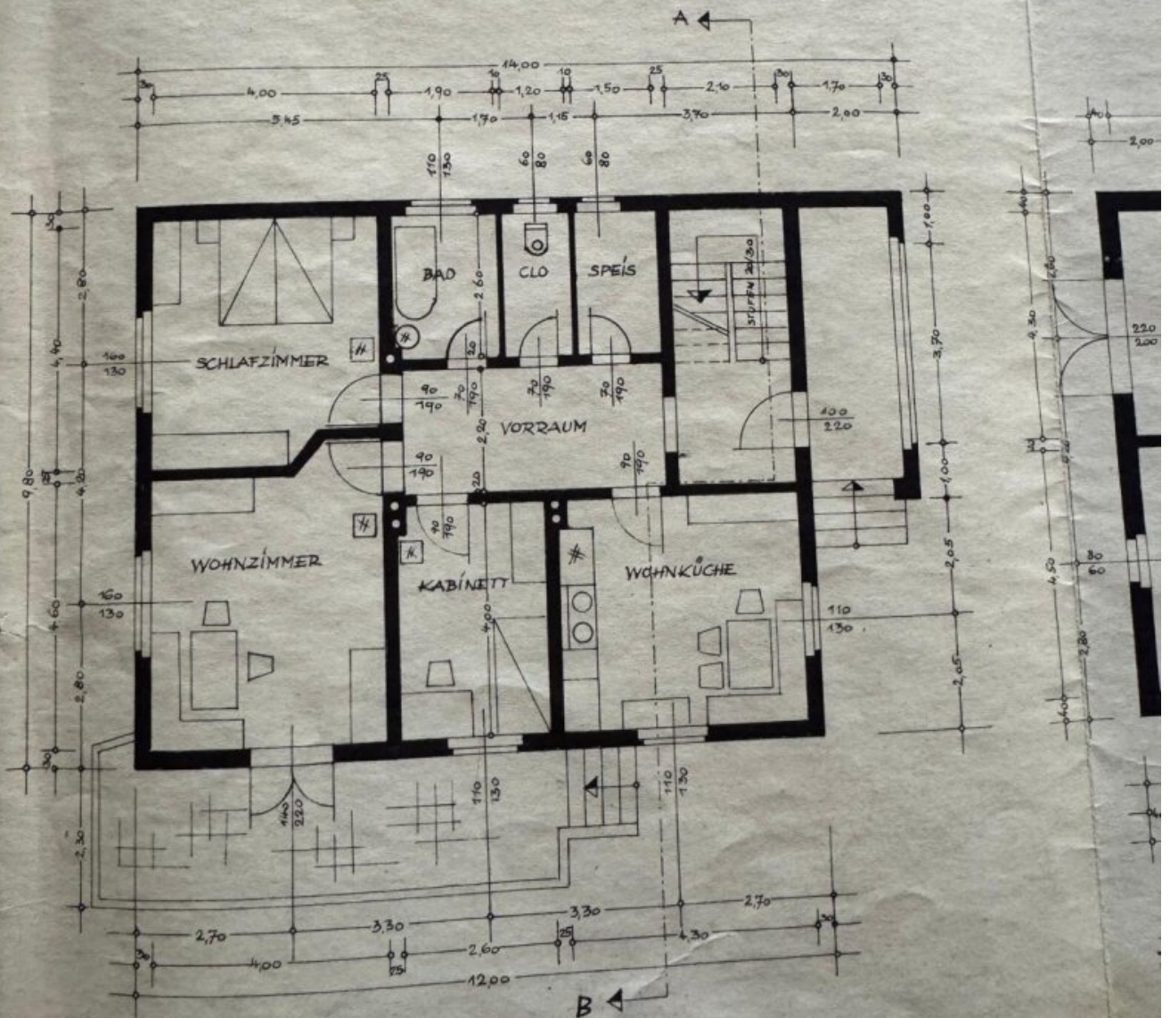
ERDGESCHOSS
