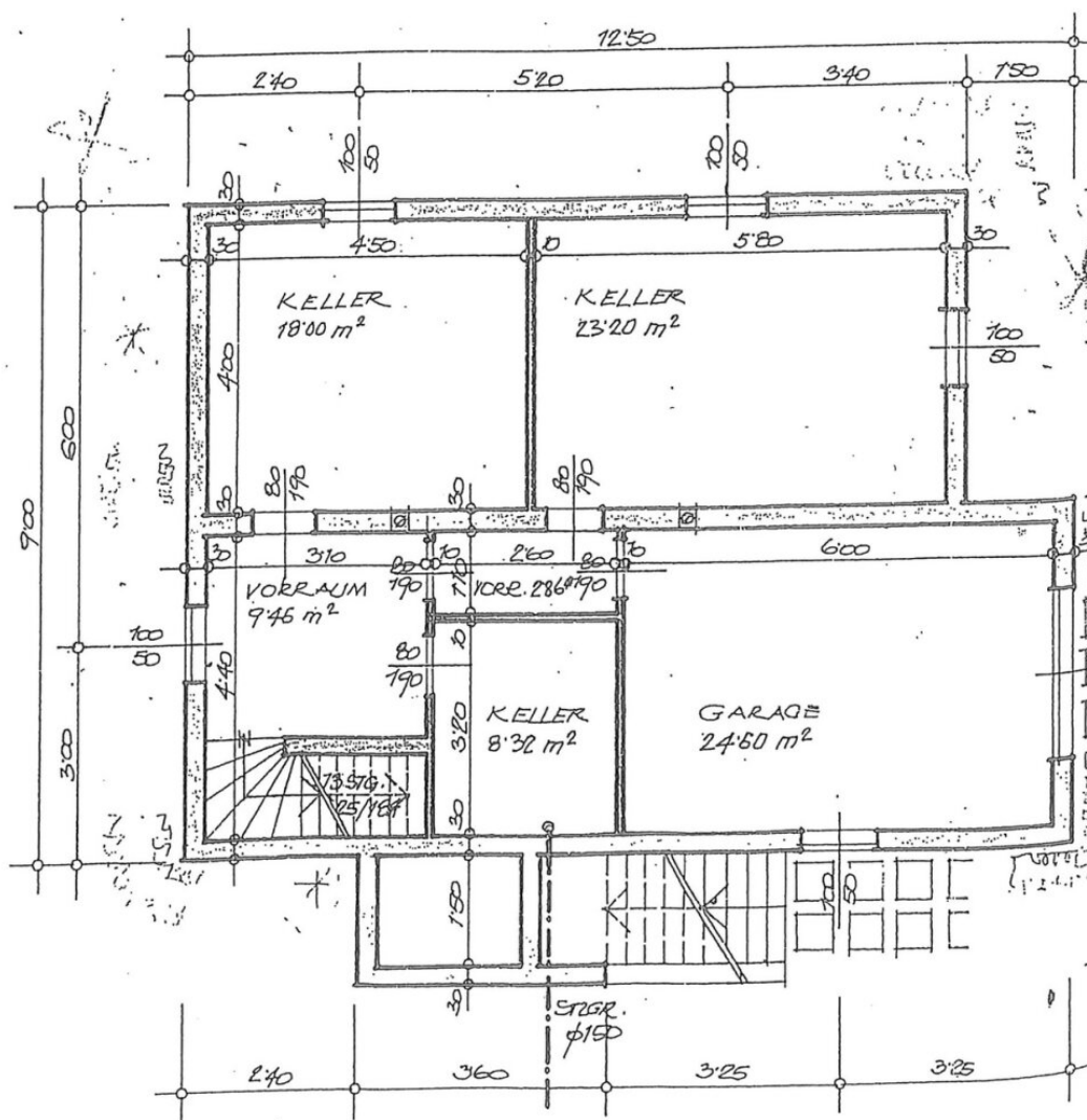
KELLERGESCHOSS
