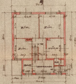
PARTERRE
