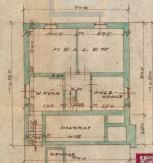
KELLER
