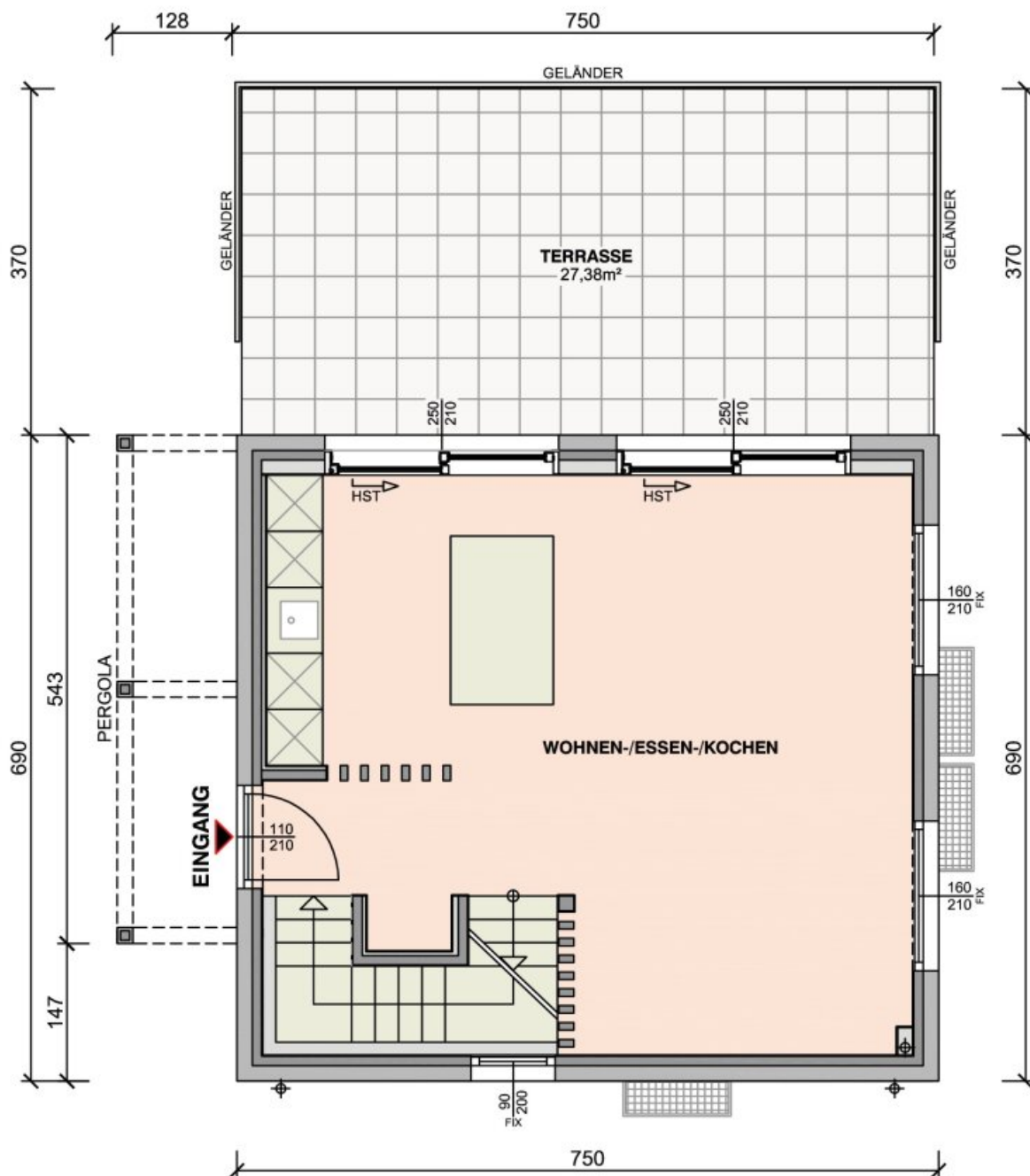
GRUNDRISS ERDGESCHOß
