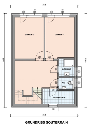
GRUNDRISS SOUTERRAIN
