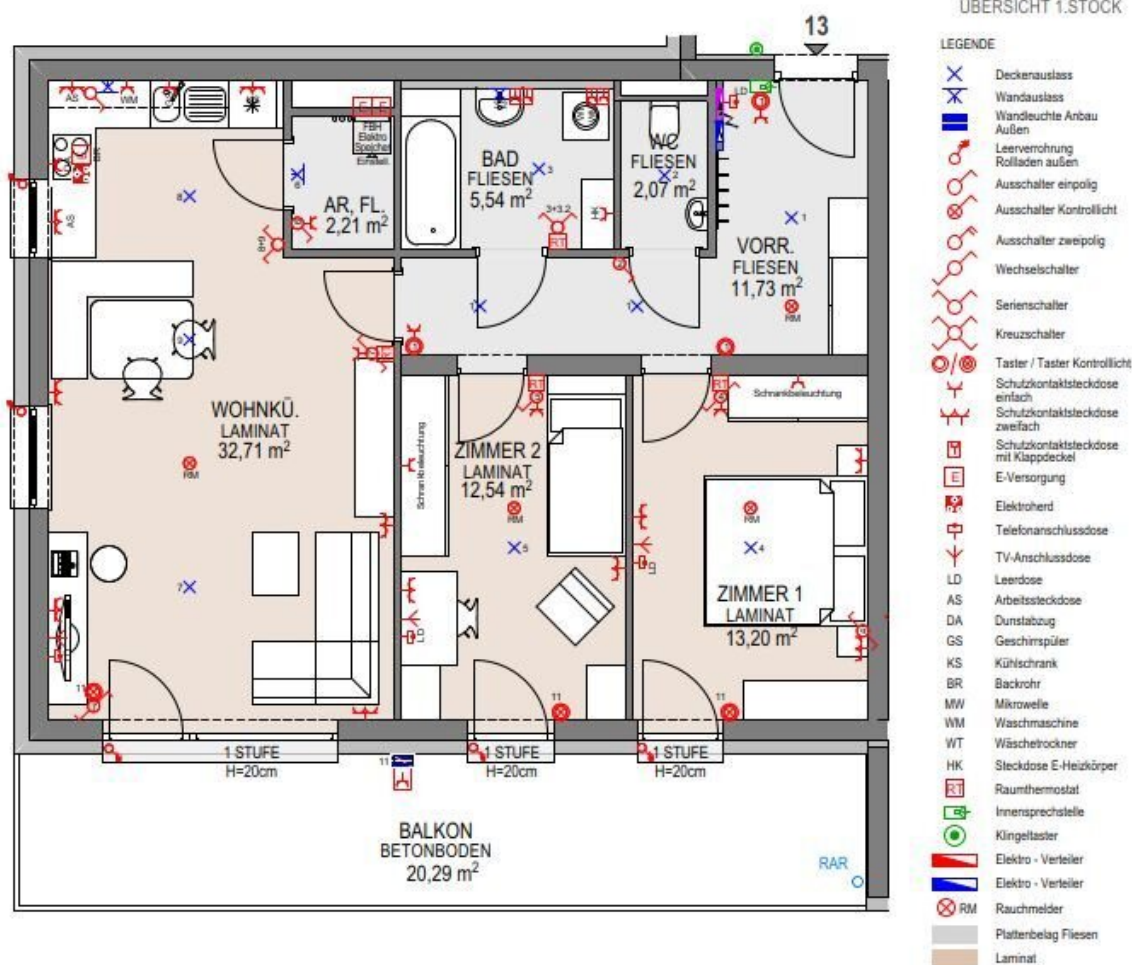
ÜBERSICHT 1.STOCK
