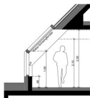
Schnitt 1
