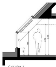
Schnitt 1
