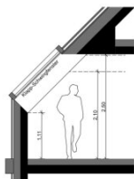
Schnitt 1
