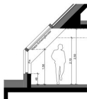
Schnitt 1
