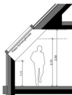
Schnitt 1
