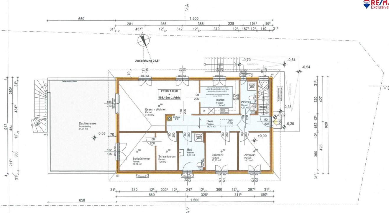
GRUNDRISS ERDGESCHOSS
