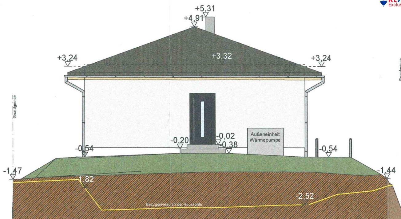
ANSICHT WEST
