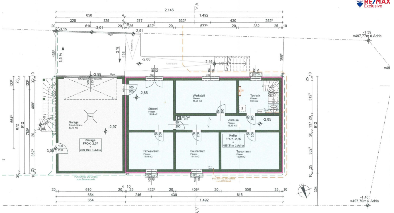
GRUNDRISS KELLER
