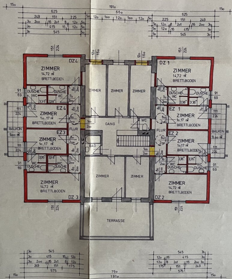
OBERGESCHOSSGRUNDRISS
