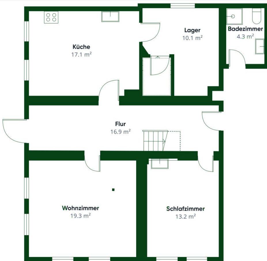
Etage 0
