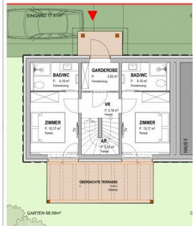
ERDGESCHOSS M 1:100
