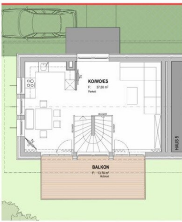
OBERGESCHOSS M 1:100
