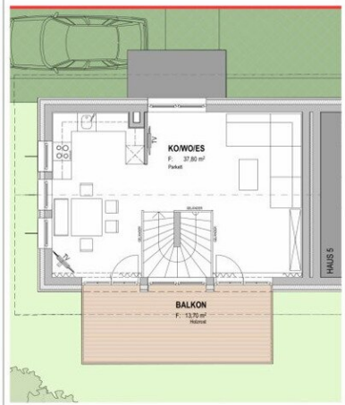
OBERGESCHOSS M 1:100
