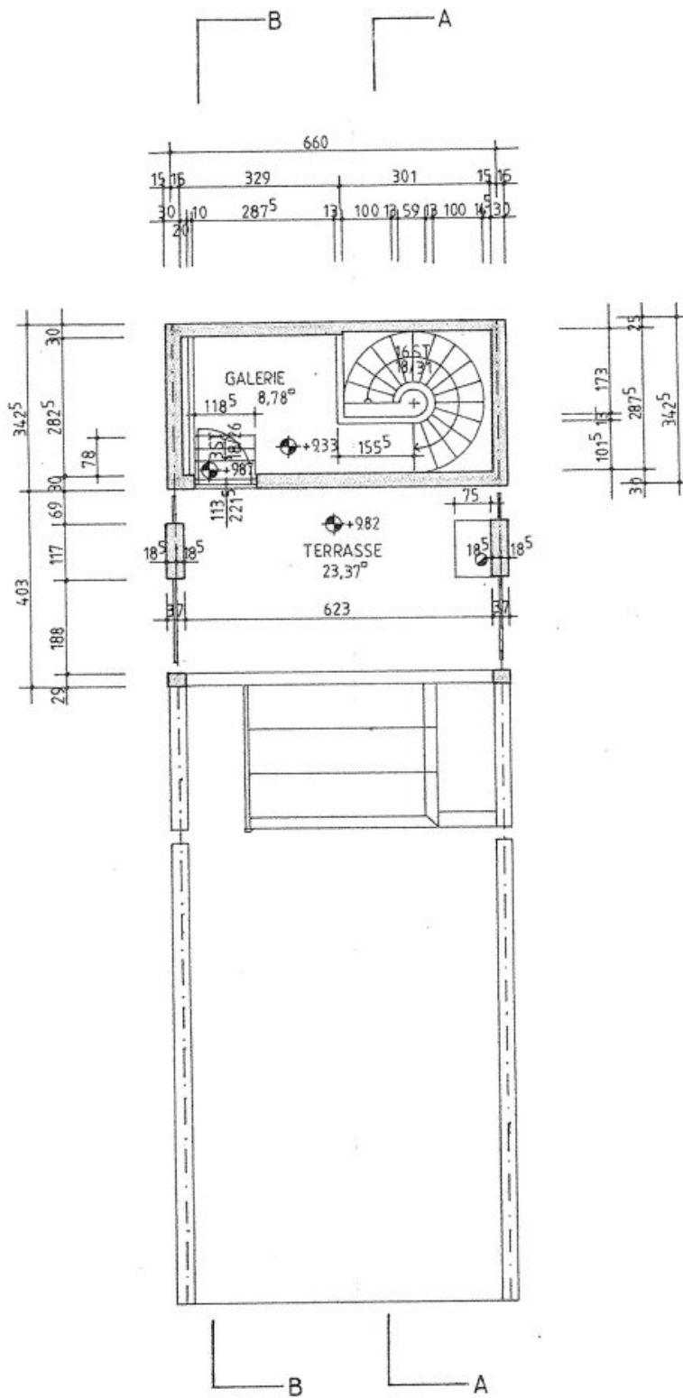
TYPI DACHGESCHOSS
