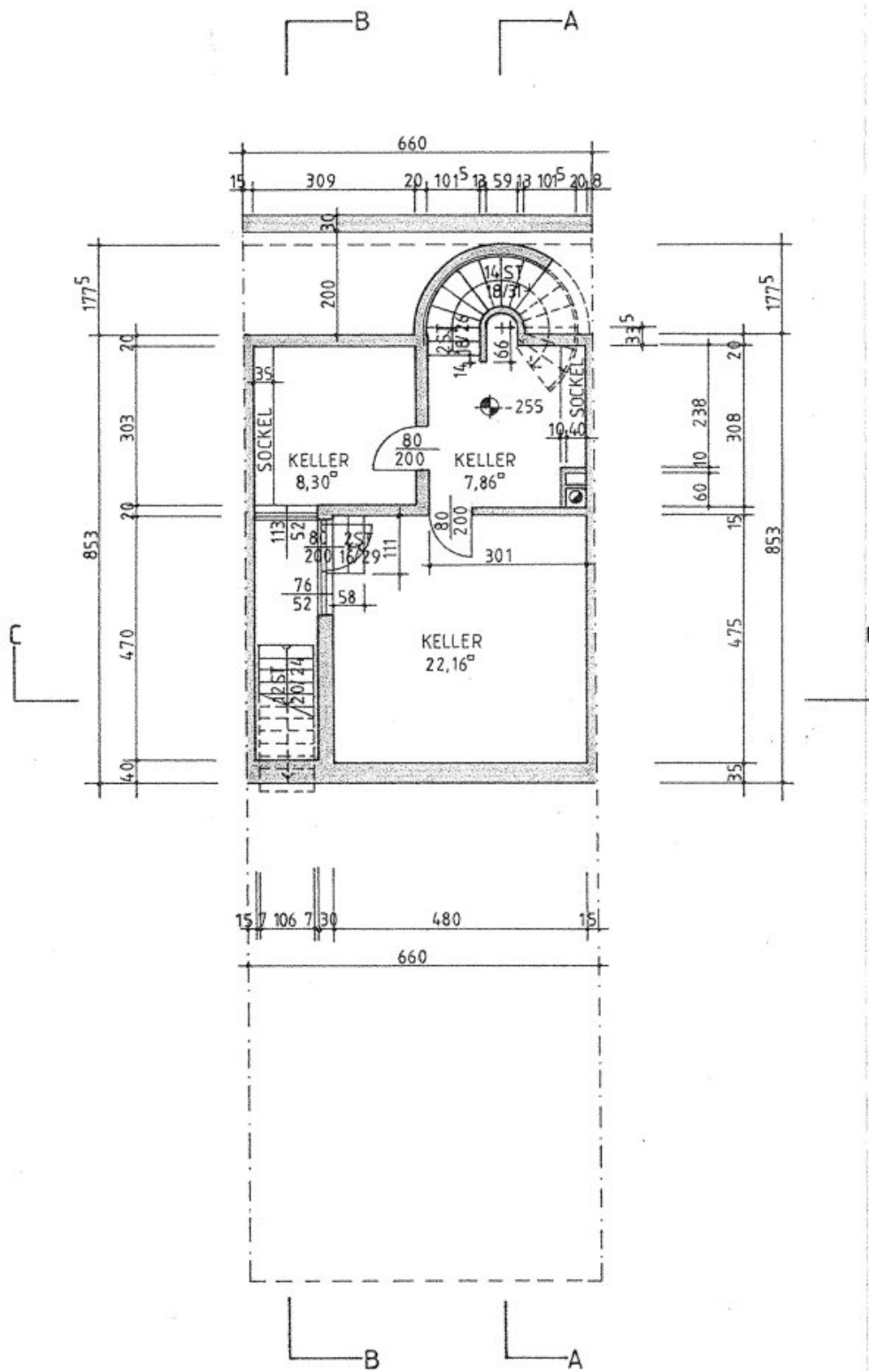
TYPI KELLERGESCHOSS
