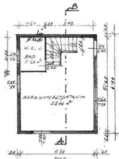
GRUNDRISS
