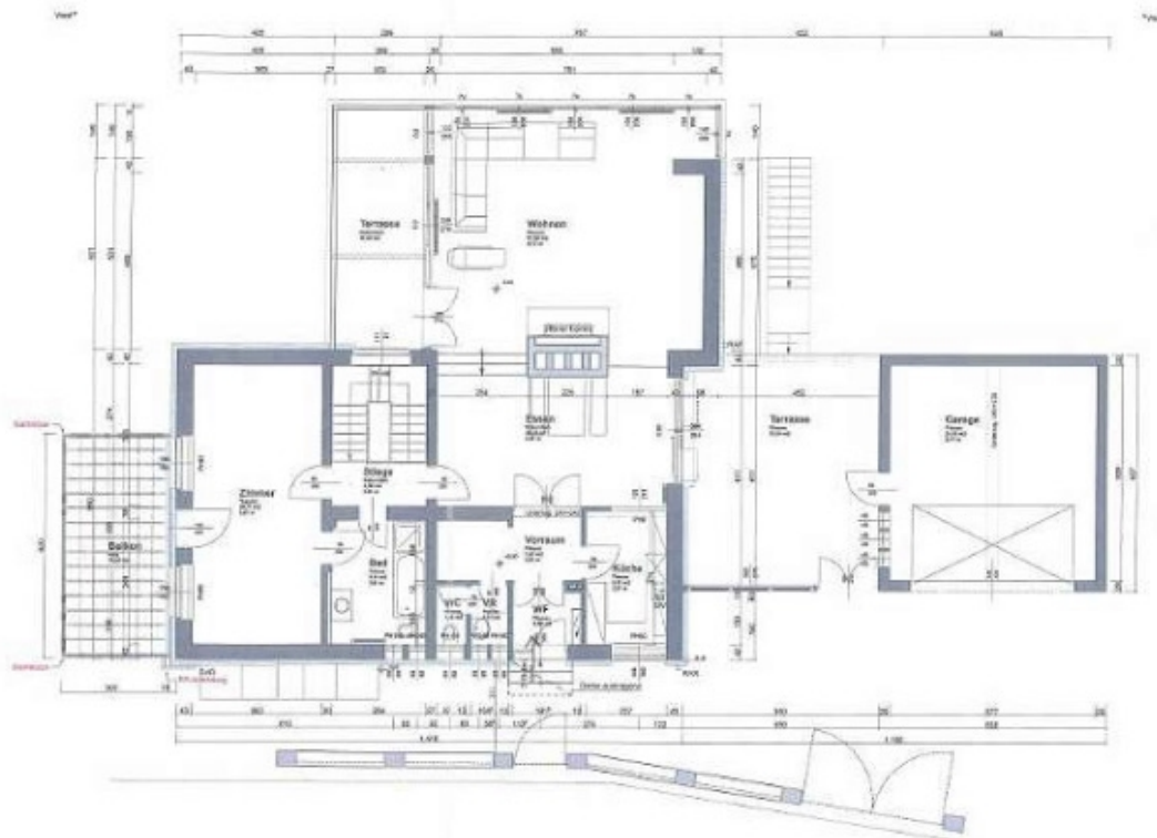
M 1:100 Erdgeschoss
