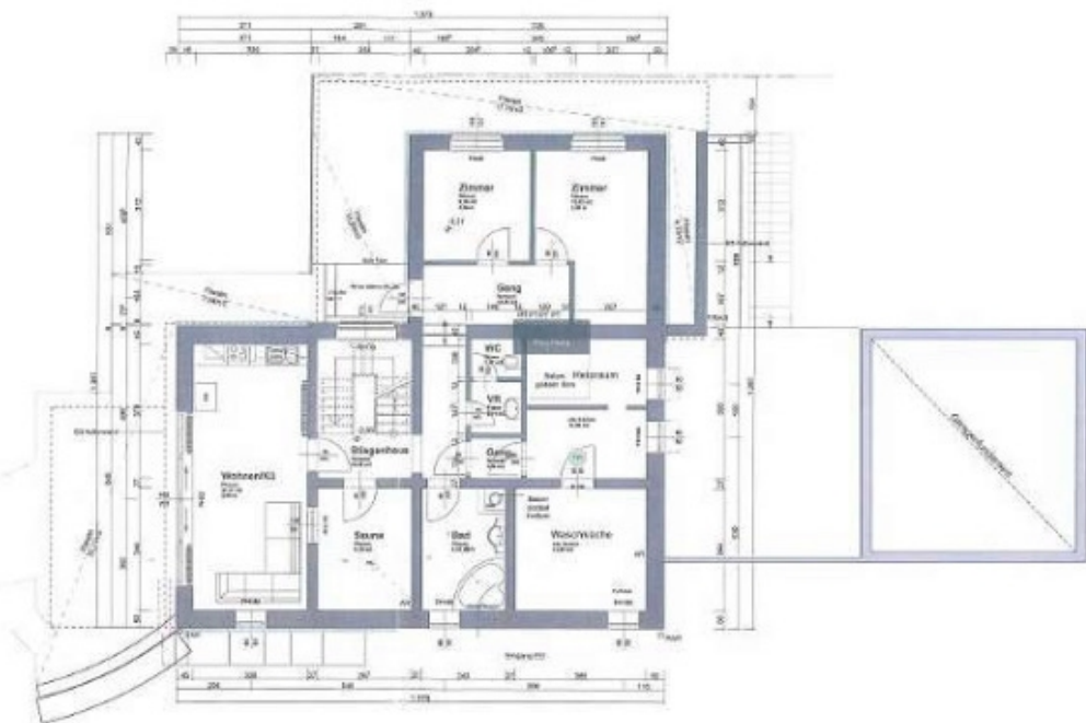
M 1:100 Untergeschoss
