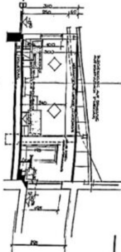
SÜDANSICHT 1/100
