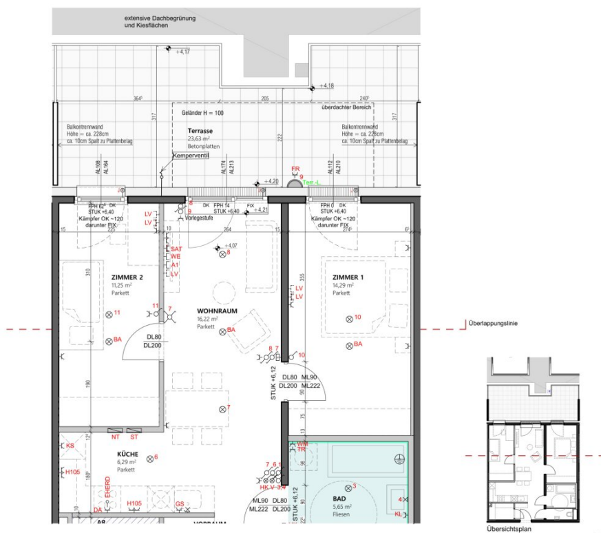
Übersichtsplan
