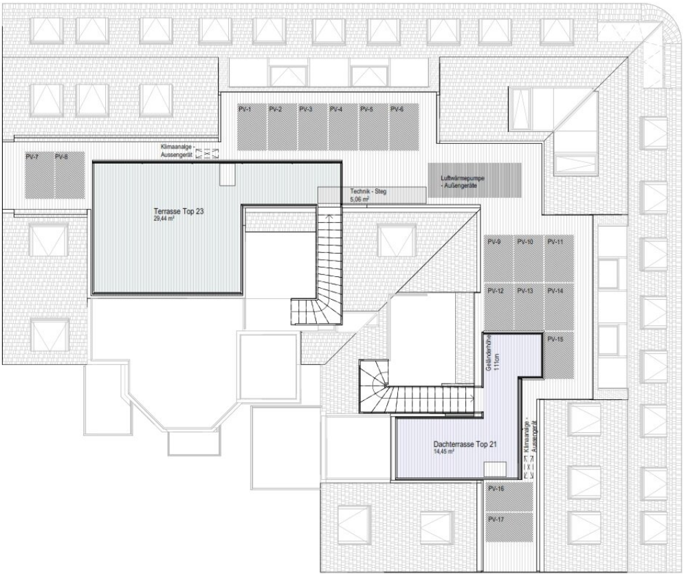
DACHDRAUFSICHT
